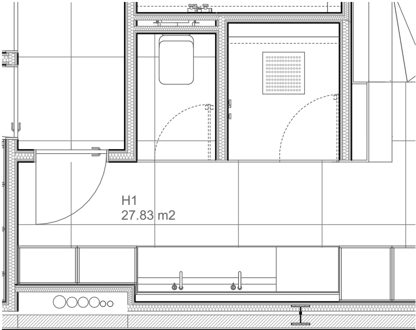
PLANTA PRIMERA FIRST FLOOR
