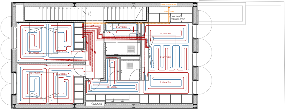
PLANTA PRIMERA FIRST FLOOR
