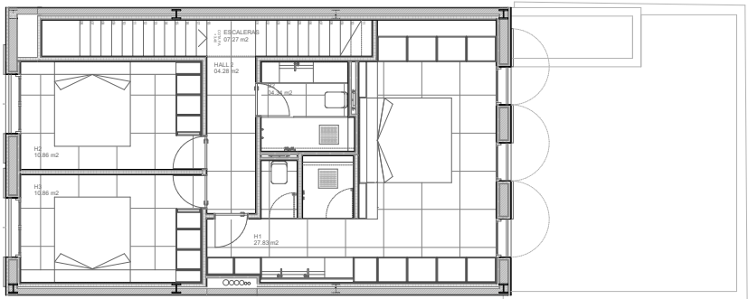
PLANTA PRIMERA FIRST FLOOR
