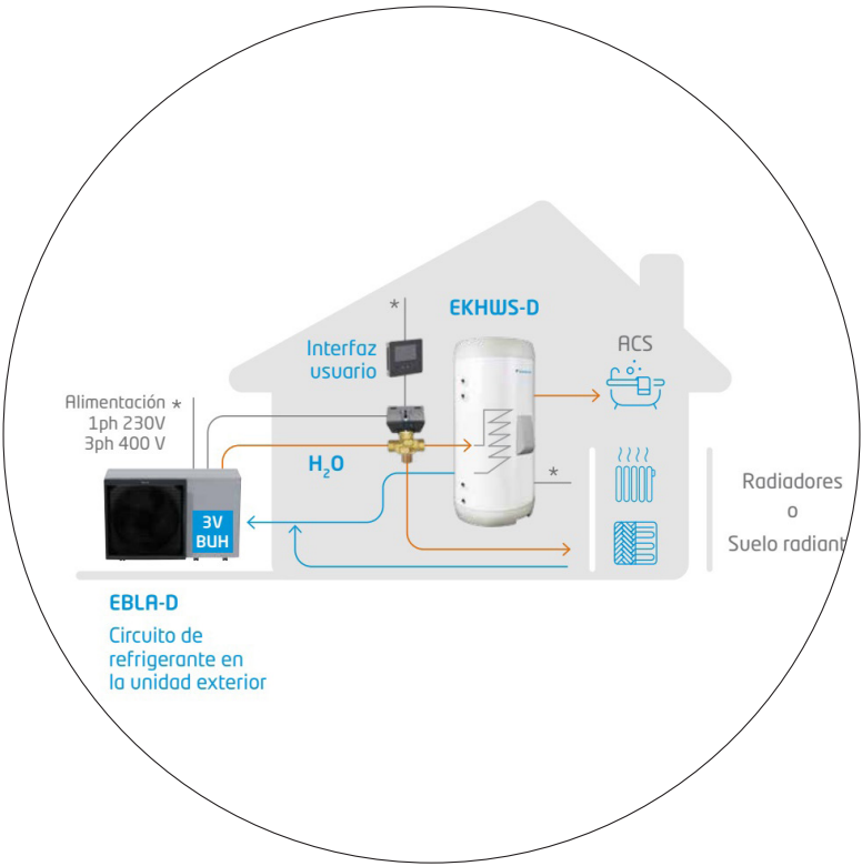
AEROTERMIA SISTEMA DAIKIN ALTHERMA 3 MONOBLOC
