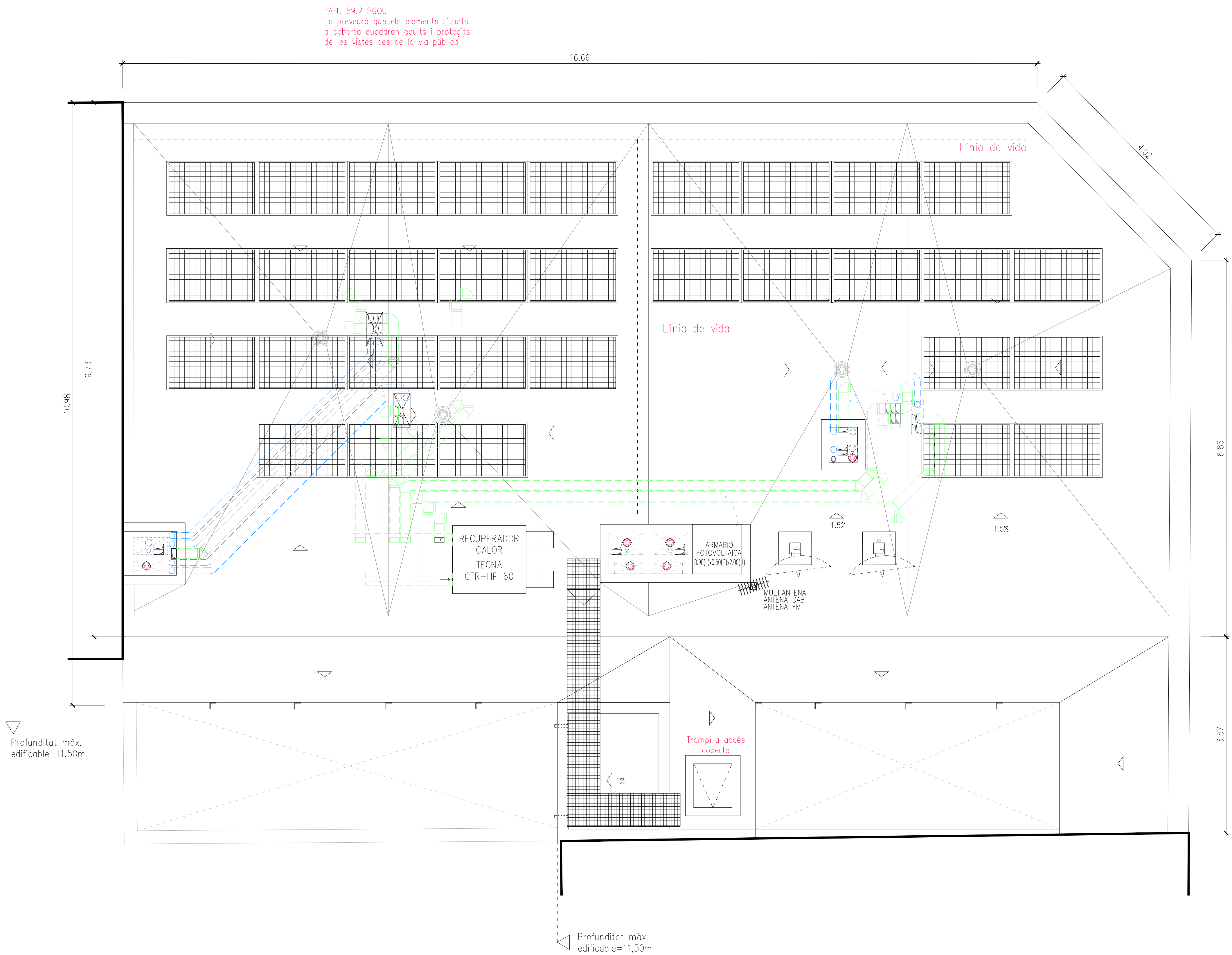
1 PLANTA COBERTA
